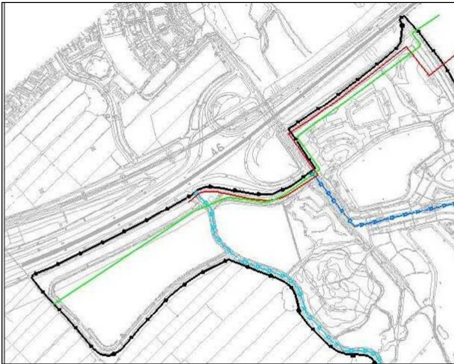
Figuur 3: Kabels en Leidingen in het plangebied.
