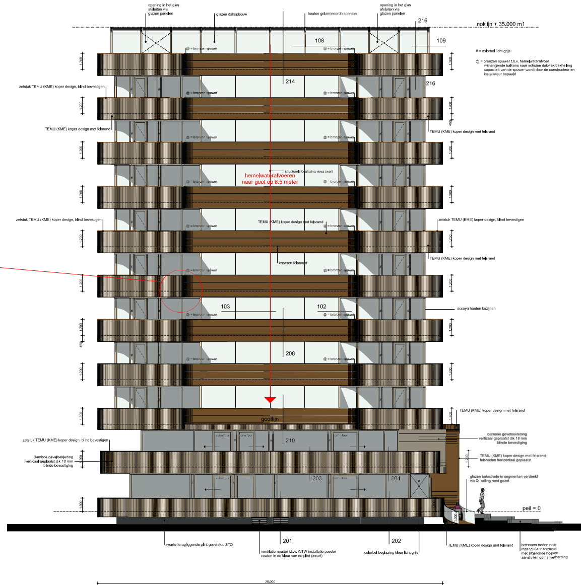
LINKERZIJGEVEL 1:100
