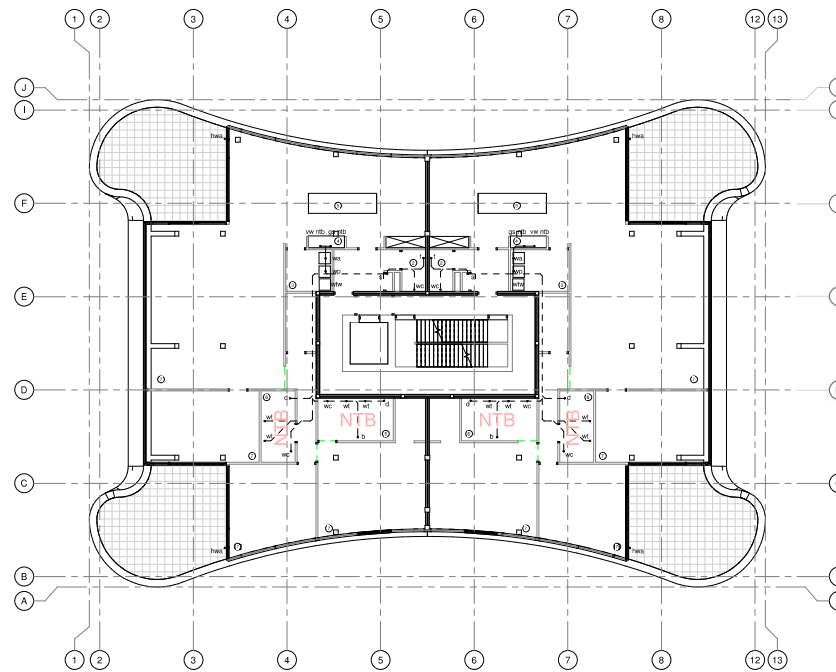
Derde Verdieping
